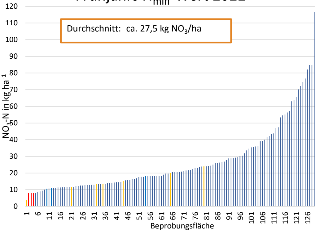
Frühjahrs N_{\min} -Wert 2022
